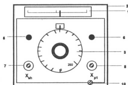
Rys.5.9. Widok przedniego panelu regulatora temperatury
