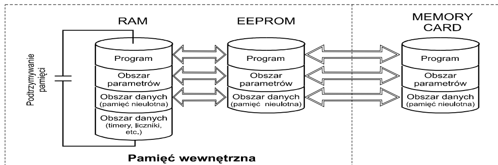
Rys. 7.11. Pamięć sterownika S7-200
