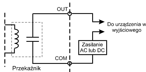
Rys. 7.4. Schemat pojedynczego obwodu układu wyjść przekaźnikowych
