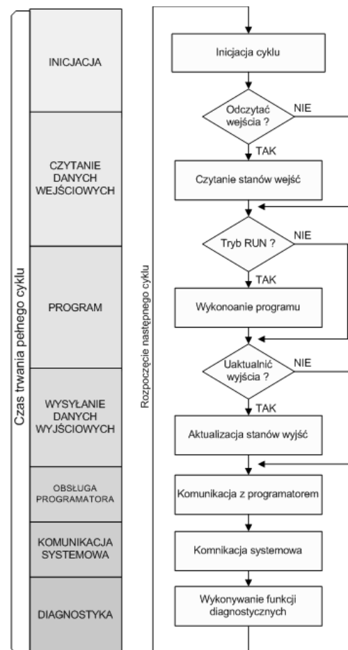
Rys. 7.2. Fazy cyklu pracy sterownika PLC
