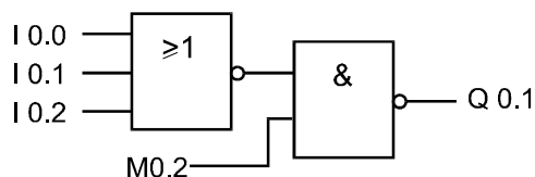
Rys.4.8. Przykładowa aplikacja zrealizowana w języku FBD
