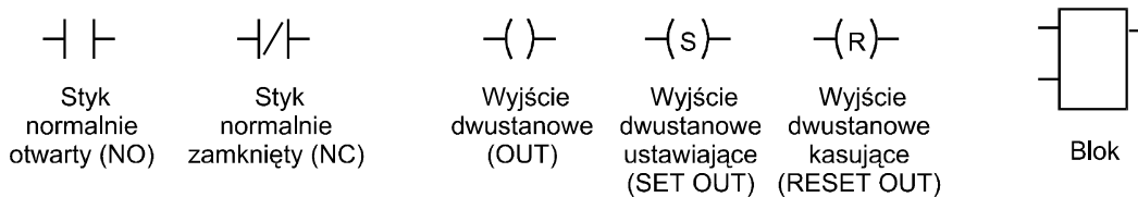
Rys.4.6. Podstawowe elementy języka LAD
