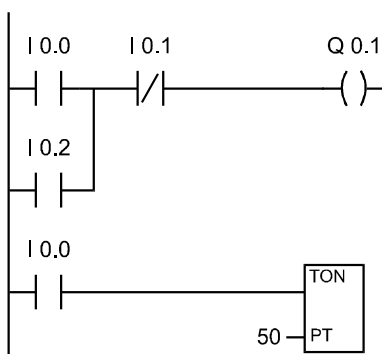
Rys.4.7. Przykładowa aplikacja zrealizowana w języku LAD
