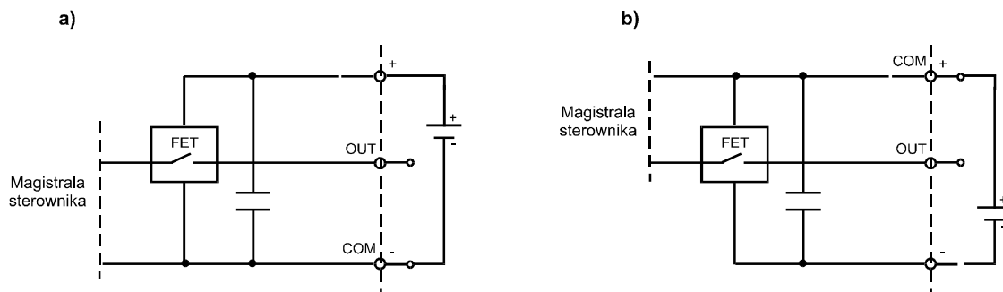
Rys. 4.5. Schemat pojedynczego obwodu układu wyjść z łącznikami tranzystorowymi: a) ze „wspólną masą” (typu źródło), b) ze „wspólnym plusem” (typu ujęcie)
