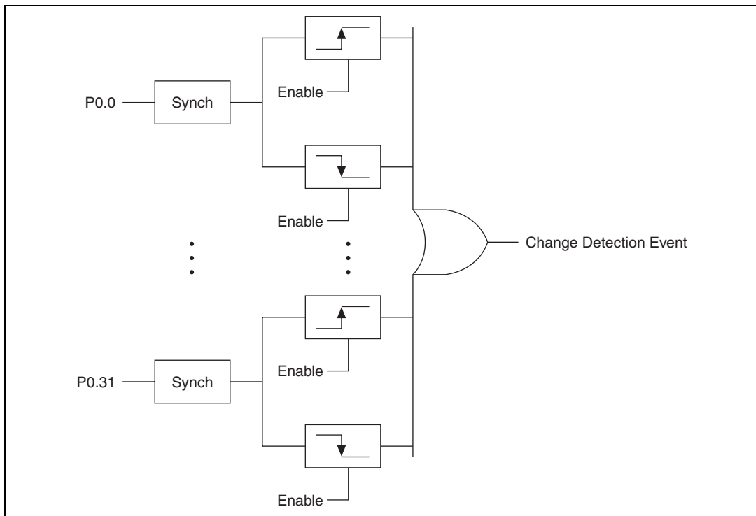
Figure 6-3. DI Change Detection
