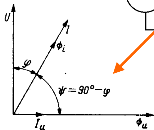
Wyidealizowany wykres wektorowy licznika indukcyjnego
