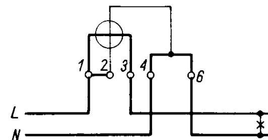
Sposób połączenia licznika jednofazowego
