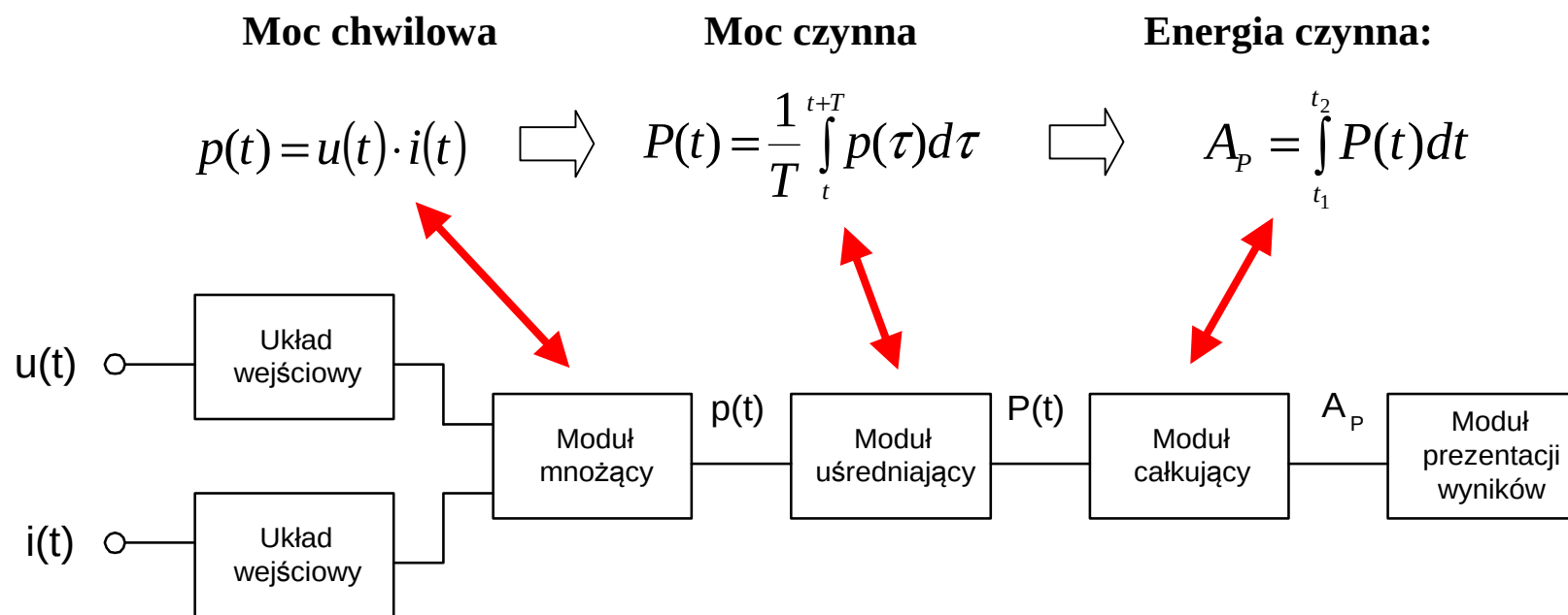
Schemat blokowy licznika energii elektrycznej
