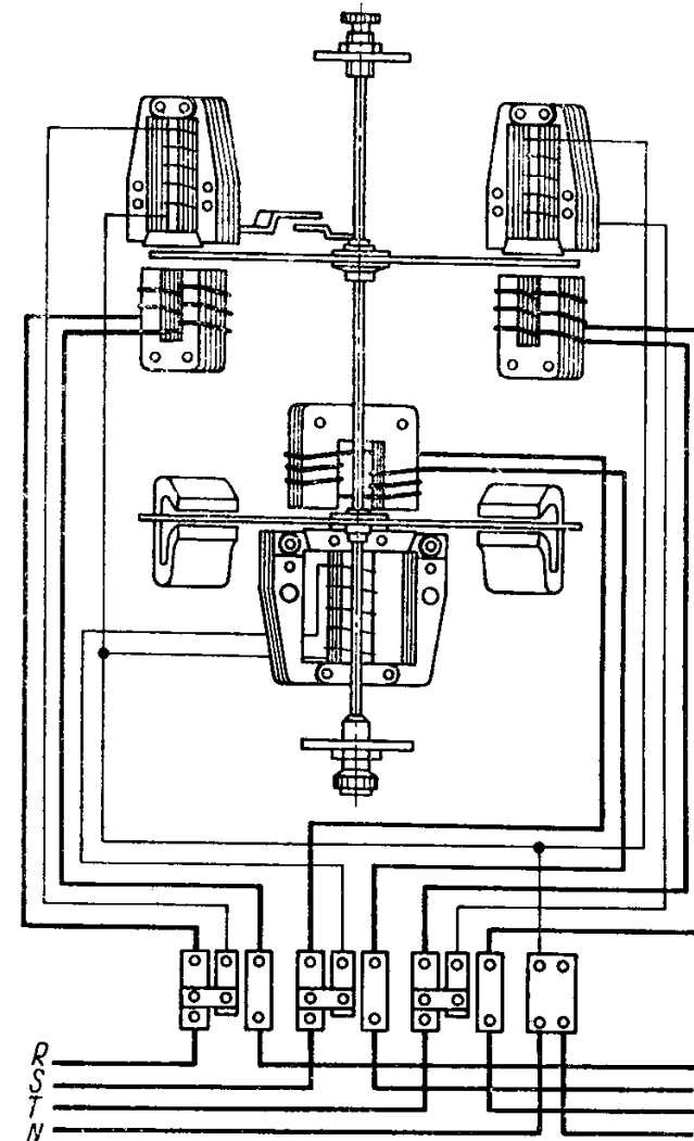
Licznik indukcyjny o trzech ustrojach
