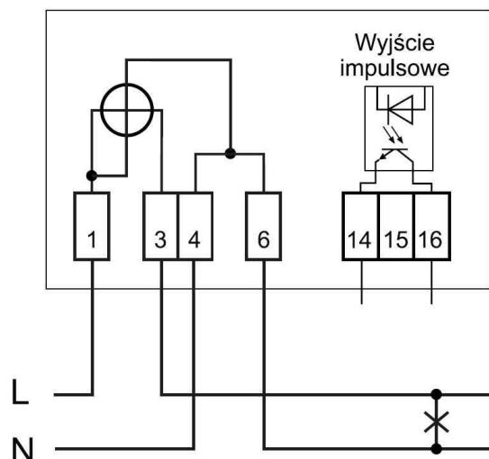
Licznik z wyjściem impulsowym
